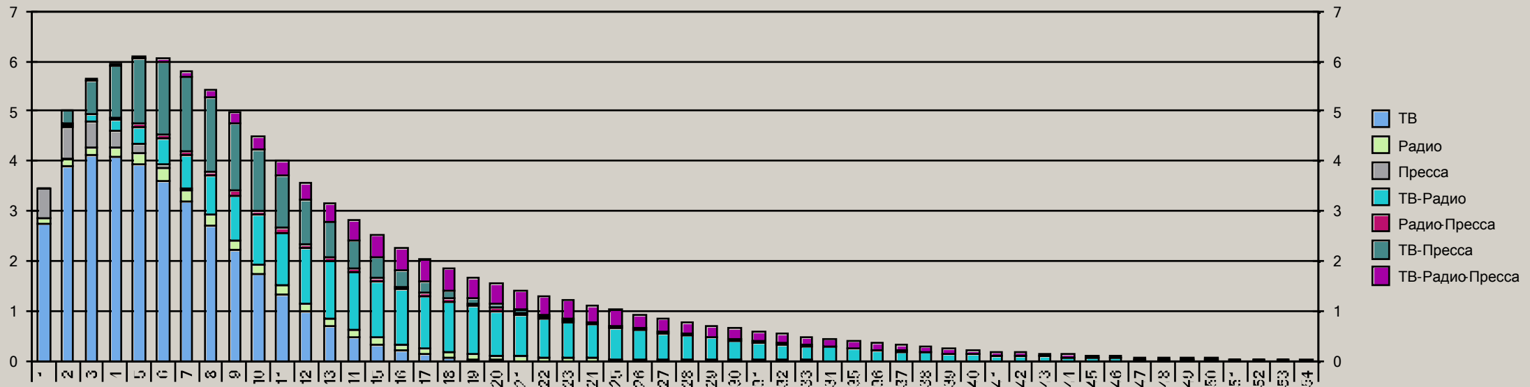
g ( f ), %
